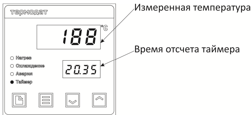
Рисунок 10 - Внешний вид прибора с включенным таймером
