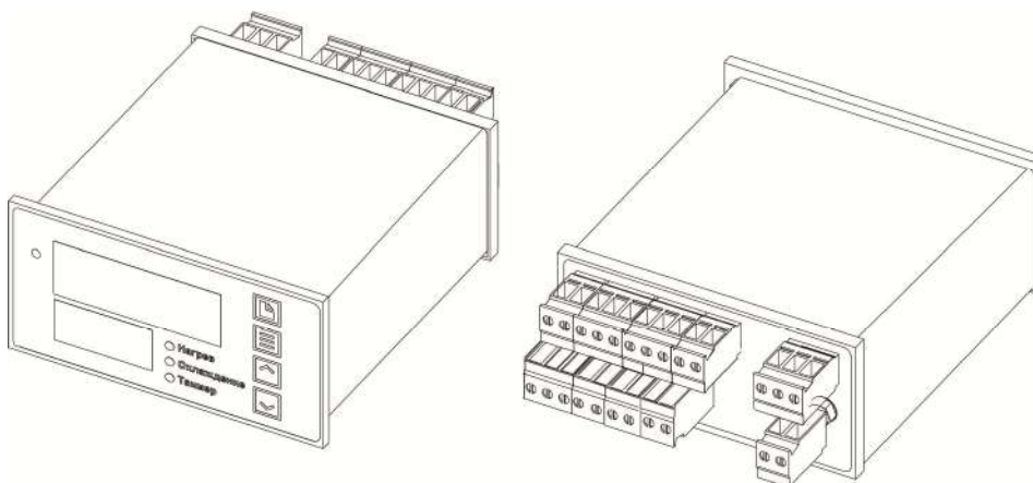
Рисунок 3 – Внешний вид прибора Термодат-12К6-D8-H...12К6-H...
