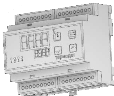
Рисунок 4 – Внешний вид прибора Термодат-12К6-P6...
